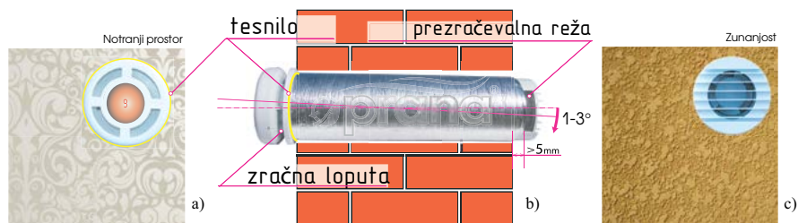
Slika 3. Shema vgradnje naprave PRANA-150, PRANA-200G, PRANA-200C v steno:
